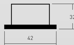
Querschnitt Versorgungseinheit
